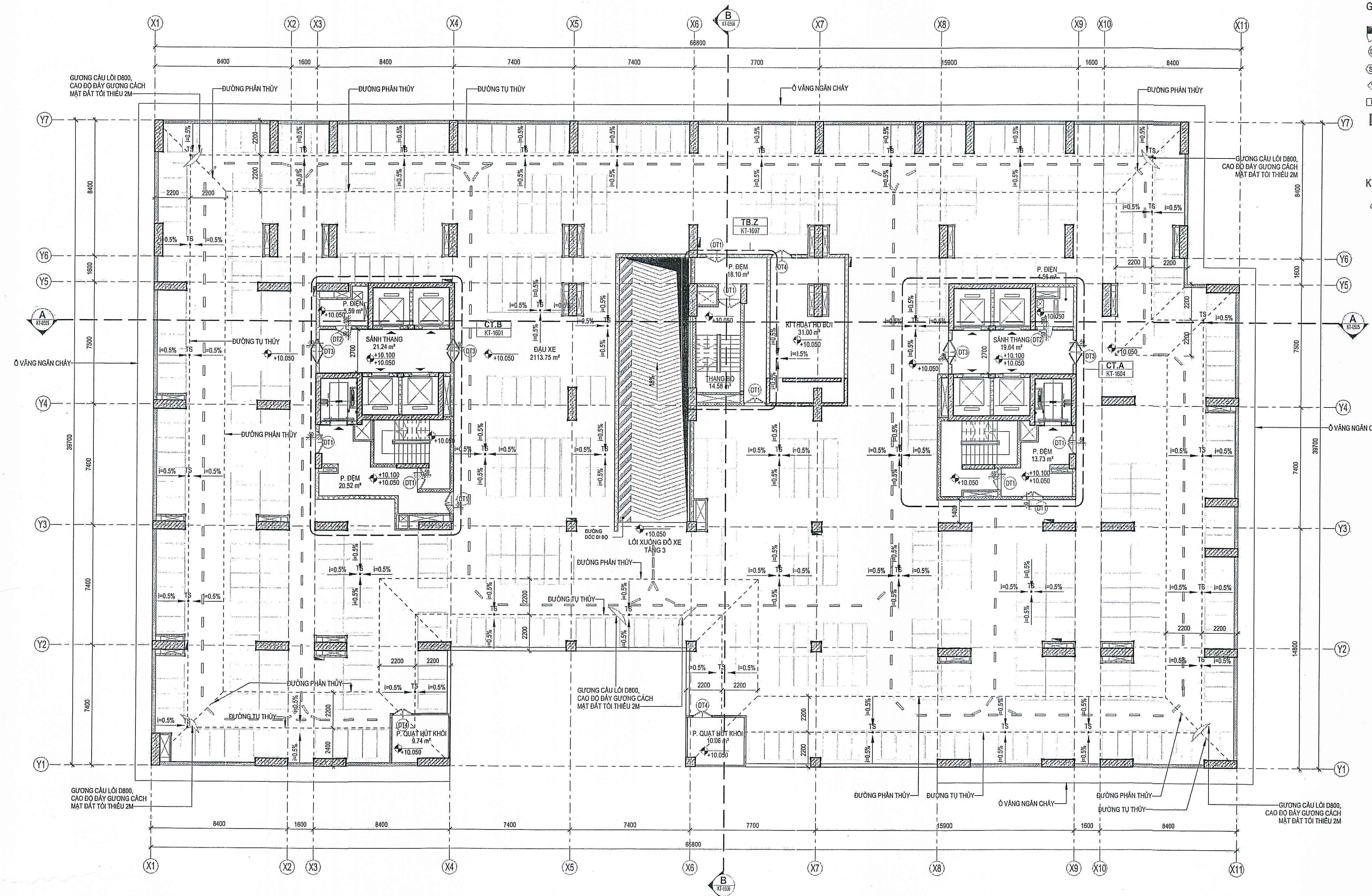
MẶT BẰNG TẦNG 4 TỶ LỆ: 1 : 150
